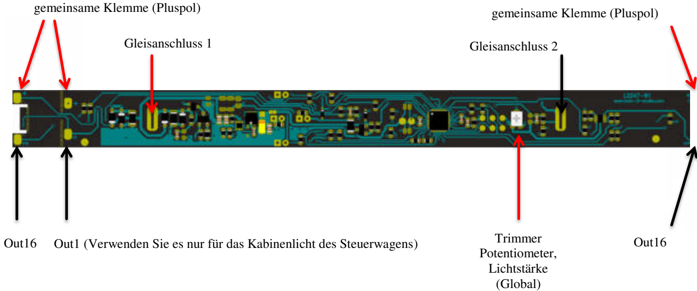
Leiterplattenansicht (Oberseite)
